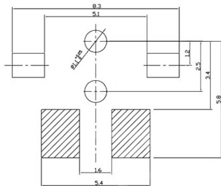
安装位置图
