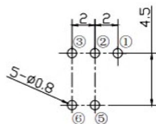
P.C.B 设计参考尺寸
