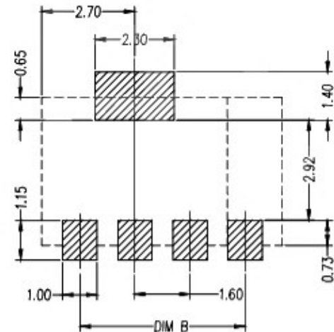
3&4PIN LAYOUT
