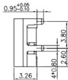
剖面图 A-A
