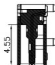
剖面图 A-A
