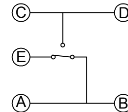
电路简图
