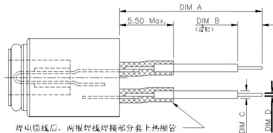
焊电缆线图
