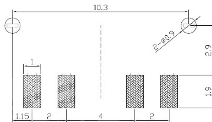
安裝圖 (PCB LAYOUT PLAN)
