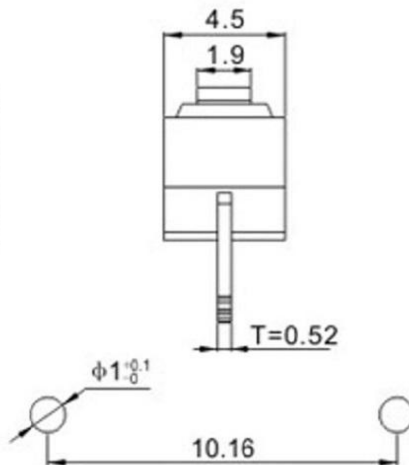
P.C.B Layout
