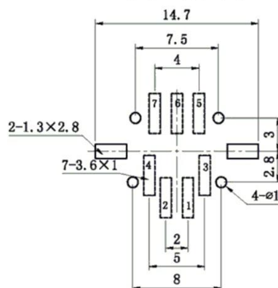
PCB板安装孔图
