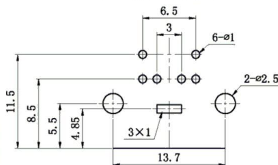
PCB板安装孔图
