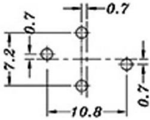
P.C.B LAYOUT
