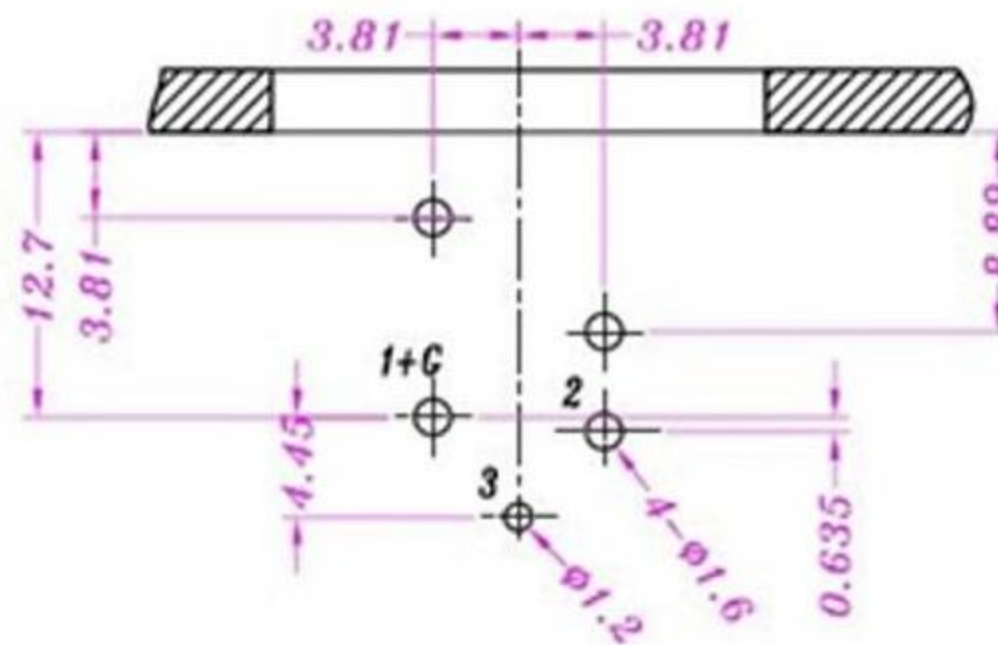
P.C.B LAYOUT
