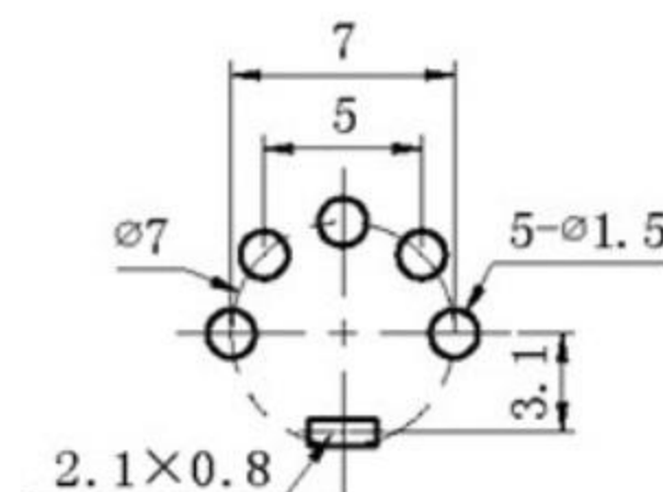
PCB板安装孔图
