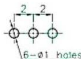
PCB Layout(Pattern Side)
