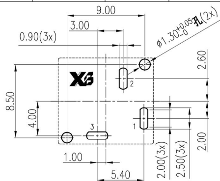
P.C.B LAYOUT(TOLERANCE: ±0.05mm) TOP VIEW(T=1.60mm)
