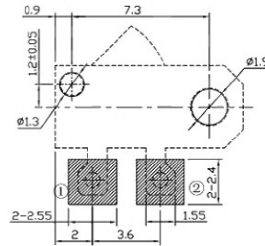
安装位置图
