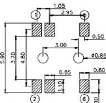
安装尺寸
