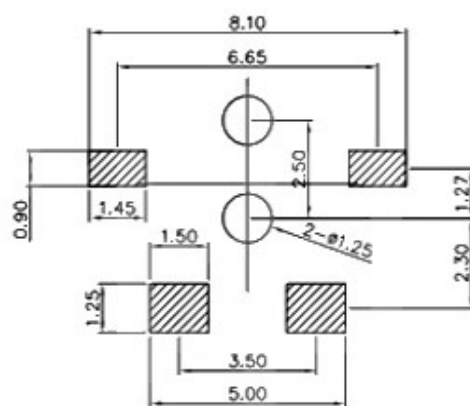
安装尺寸
