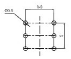
印刷电路板 Recommended P.C.B Layout
