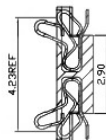
剖面 A-A
