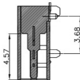
剖面图A-A
