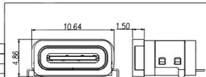
加防水圈示意图
