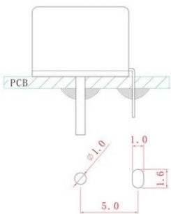
PCB焊锡插脚孔位
