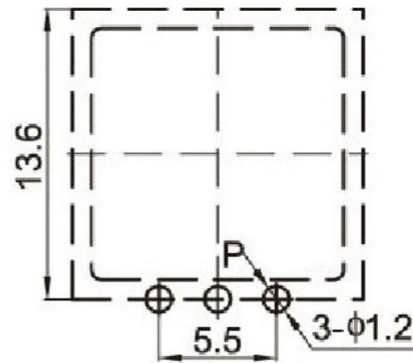
印制线路板 P.C.B
