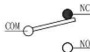
电路图
