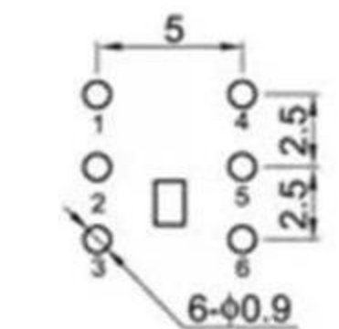
印制电路板 printed-circuit board
