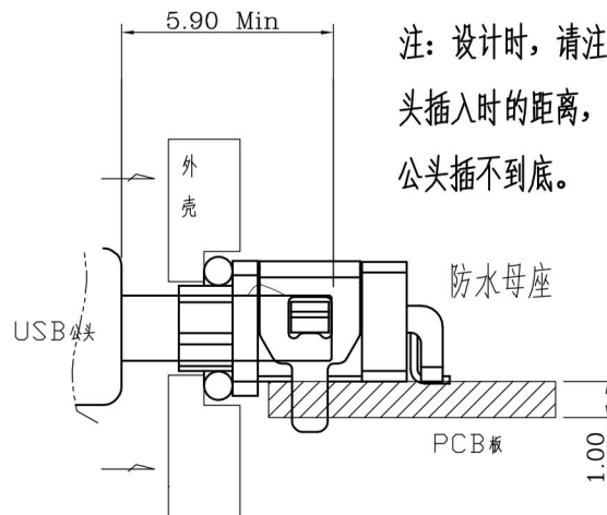
组装示意图
