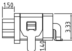
组装示意图
